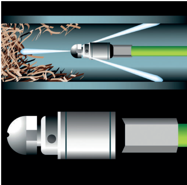
Exemple de tête de curage
